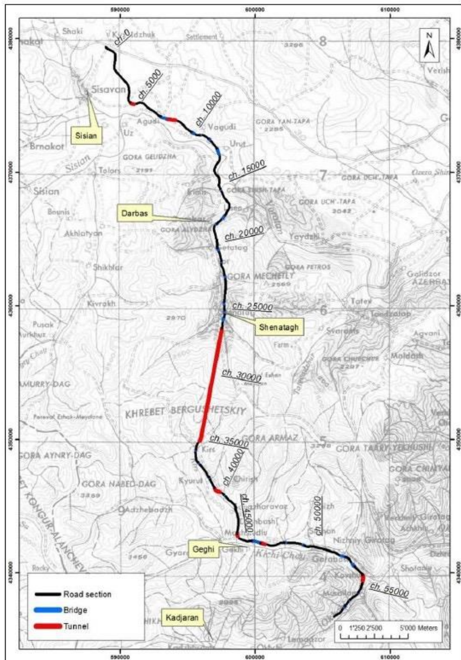
Նկ. 2. Կառուցվող Միսիան-Քաջարան ճանապարհը թունելների և կամուրջների դիրքերի հետ միասին
